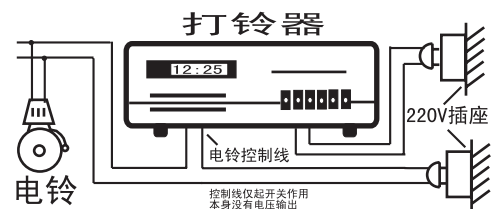
Tw833接线图
