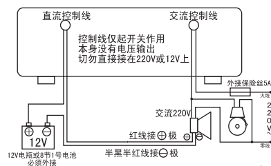
有喇叭有交流电铃的的接法
