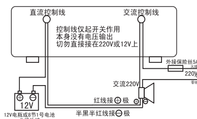
有喇叭无交流电铃的的接法
