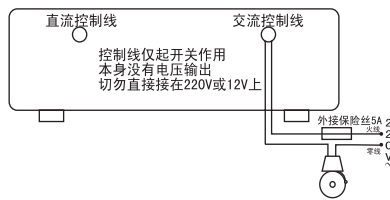
只有交流电铃的的接法
