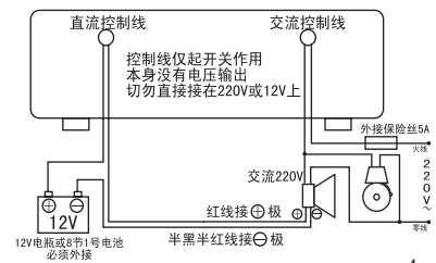
有喇叭有交流电铃的的接法
