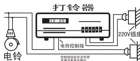
TW837接线图
