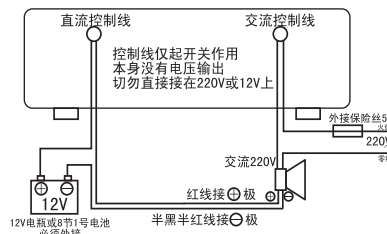
有喇叭无交流电铃的的接法
